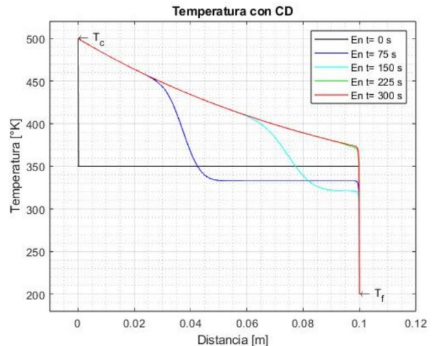
Figura 2. Evolución de temperatura en el conducto, estimada por resolución de una ecuación de transporte mediante el Método de Volúmenes Finitos.
