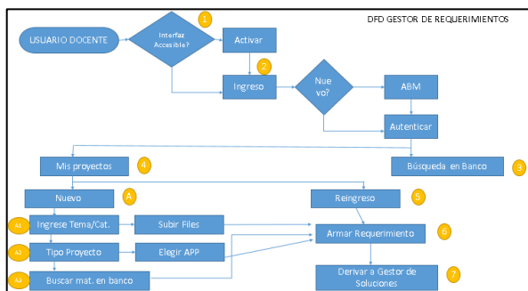
Figura 6. Diagrama de Flujo de Datos del Gestor de Requerimientos
