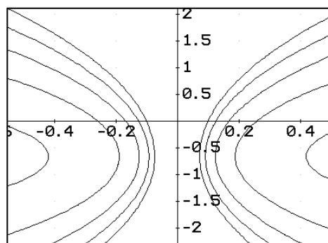
Figura 7: Gráficas de 3x^2 + 3y^2 + Cx + 4y + 5 = 0
